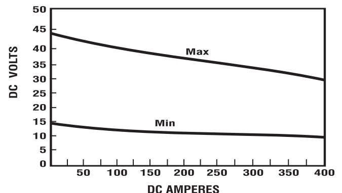
Volt - Amp Curve
